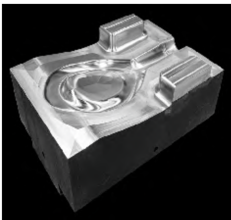
फोर्जिंग डाई
