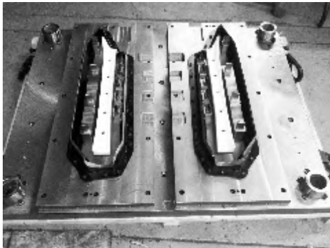
CUTTING DIE
